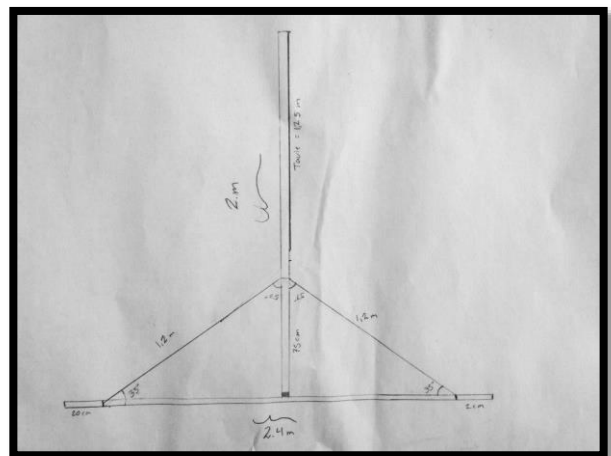
Skitse af tavlens ben fra siden, med mål og vinkler.
